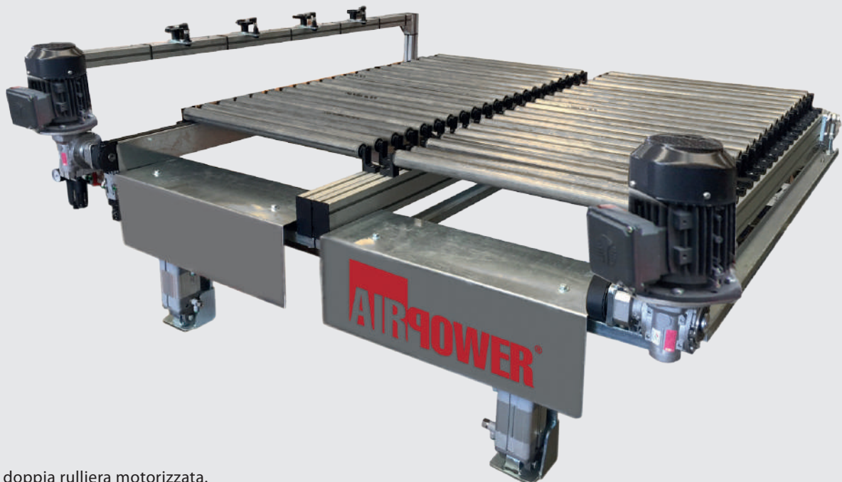
Espulsore doppia rulliera motorizzata.
